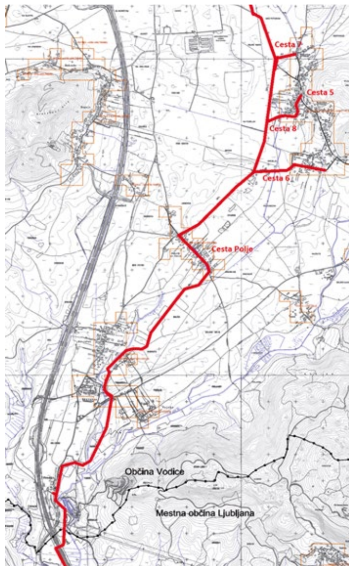
Predvidena trasa fekalne kanalizacije Projekta C0 v Občini Vodice
